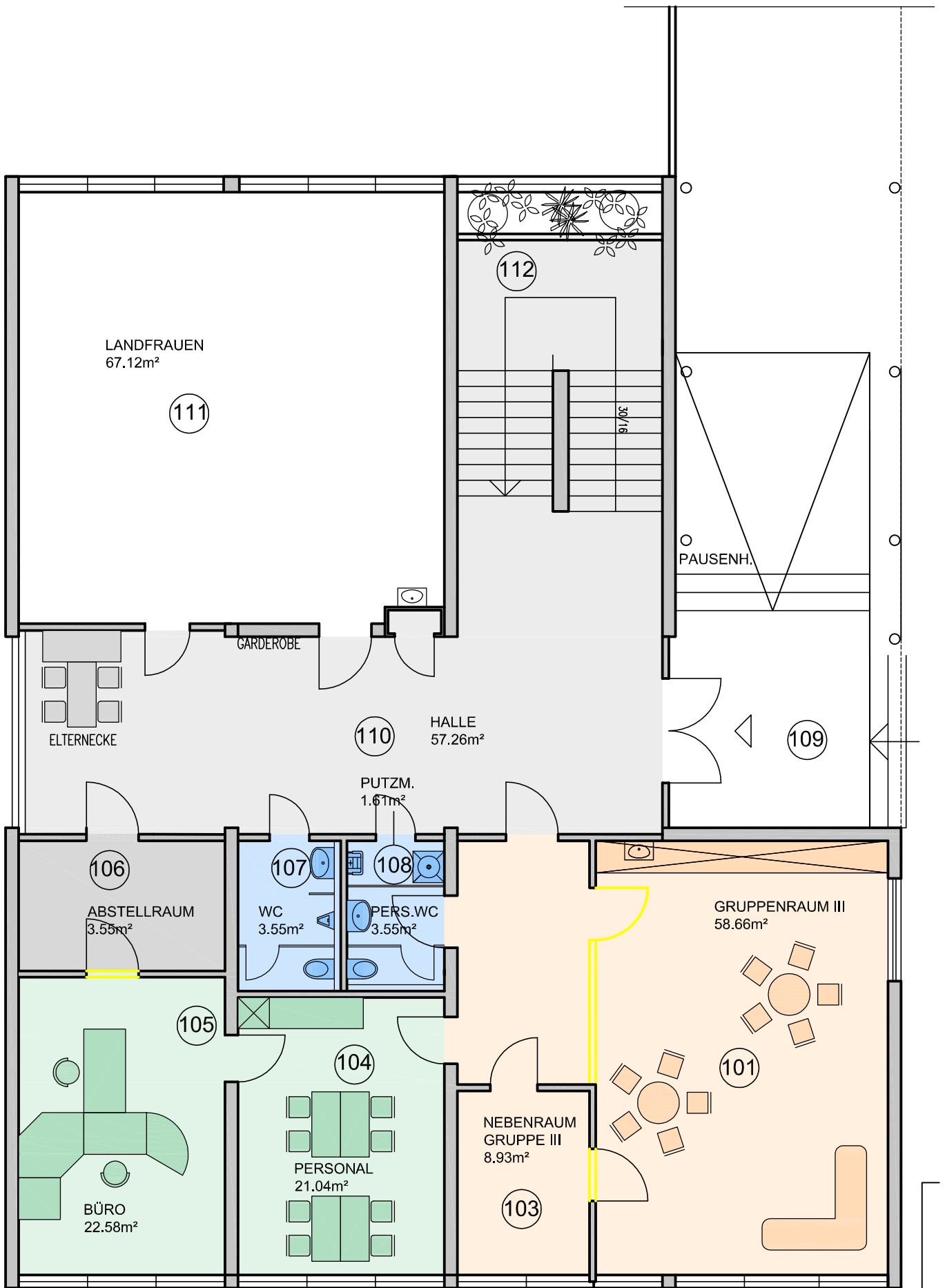
"NEUBAU" GRUNDRISS ERDGESCHOSS M 1:100
